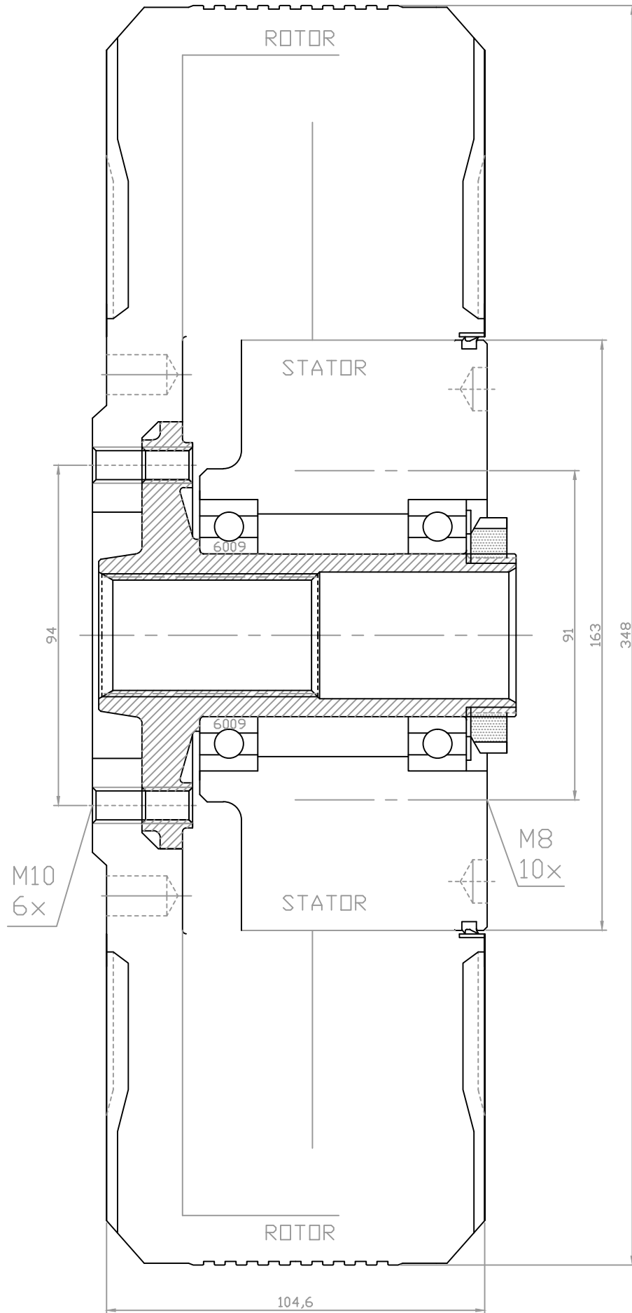
EMRAX 348 300kW_1000Nmp_39kg
